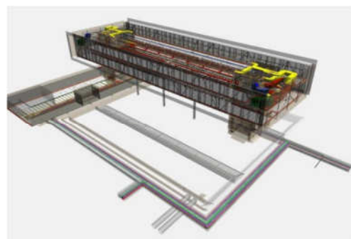
BIM modellen av design senteret, inkludert alle tekniske installasjoner som spenner fra elektro, ventilasjon, oppvarming, kjøling og sanitær.
